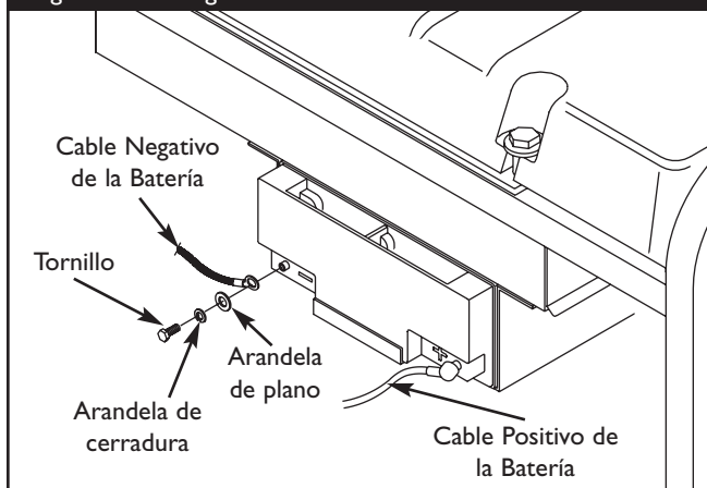
Figura 11 — Negativo Alambre las Conexiones
